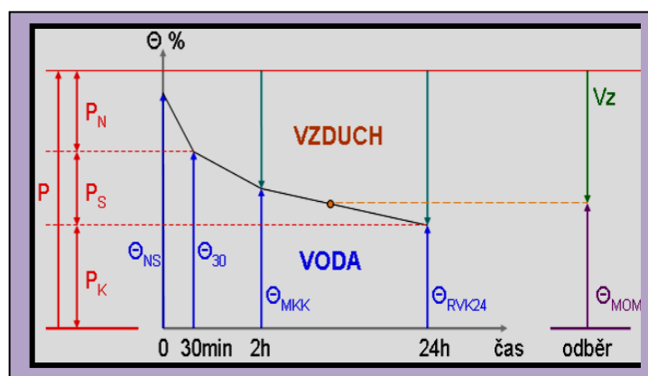
BOX 4—7: Analýza fyzikálního válečku pro stanovení půdních hydrolimitů
