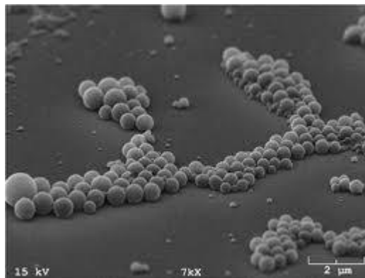
Paramagnetické částice
