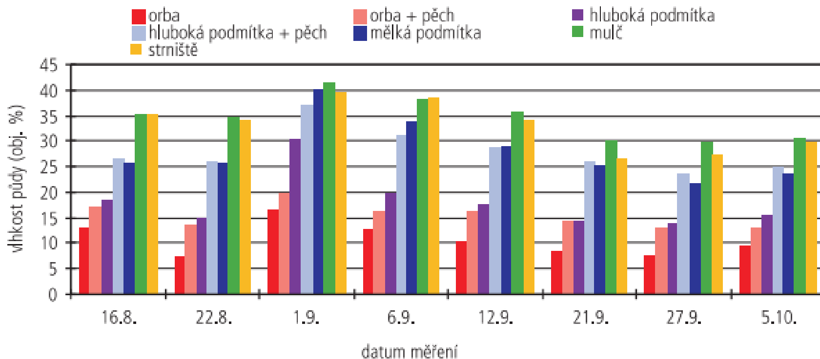
Vlhkost půdy do hloubky 12 cm při různém zpracování po sklizni ozimé pšenice (Ruzyně 2023)
